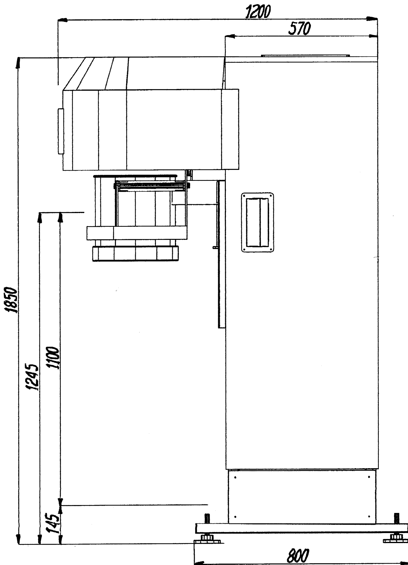
Widok z boku dozownika do worków otwartych wraz z wymiarami ( wersja z uchwytem pneumatycznym )
