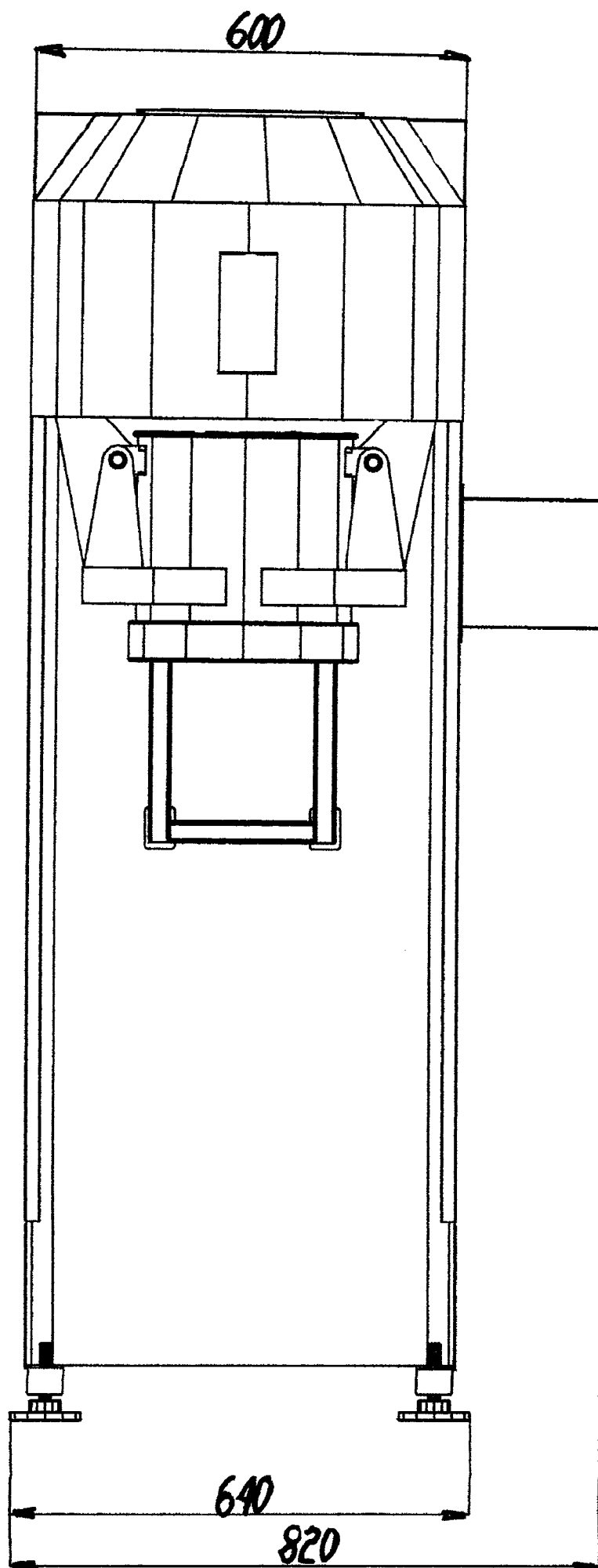
Widok z przodu dozownika do worków otwartych wraz z wymiarami ( wersja z uchwytem pneumatycznym )
